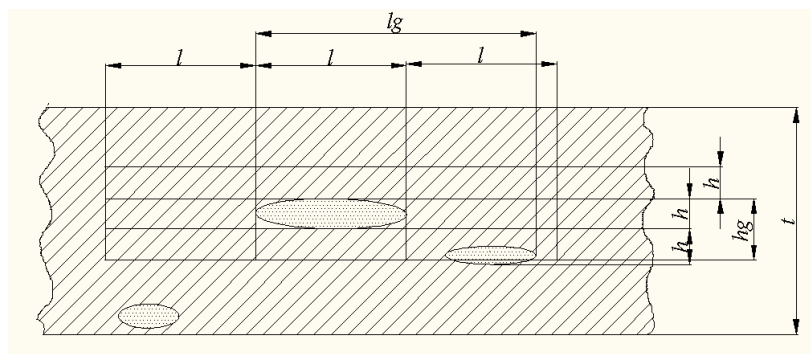
Figure 6.4.2.2 Grouped Flaws
