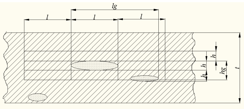
Figure 6.4.3.2 Grouped Flaws
